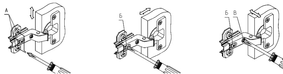
Схема 4. Регулировка зазоров и положения фасада
