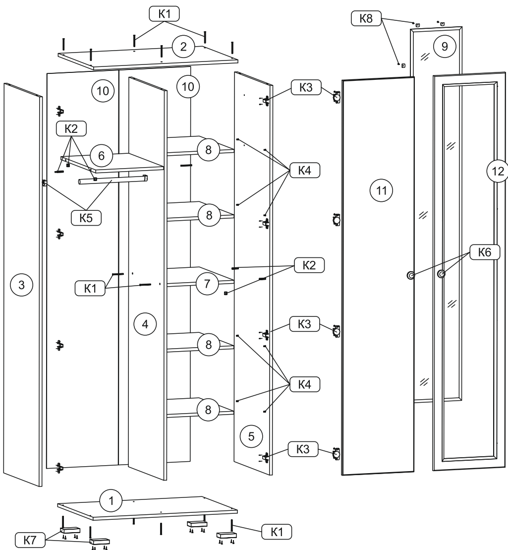
Схема 1. Сборка шкафа
