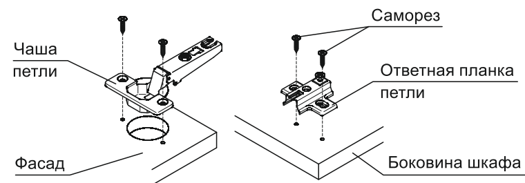
Схема 3. Установка петли
